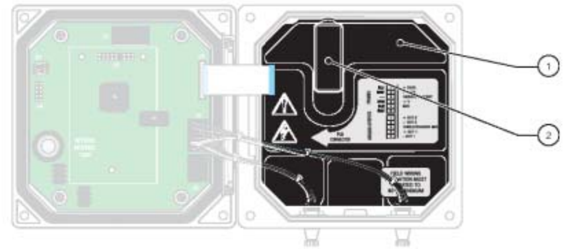
图 3-11 去掉高压隔离板
